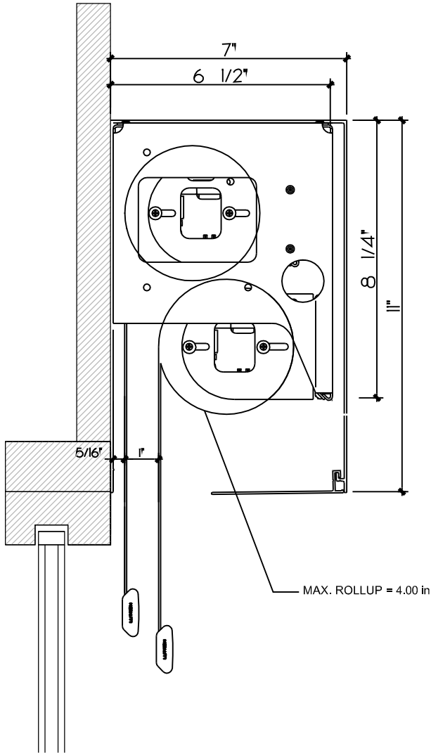
BRACKET SECTION SCALE: 3"=1'-0"
